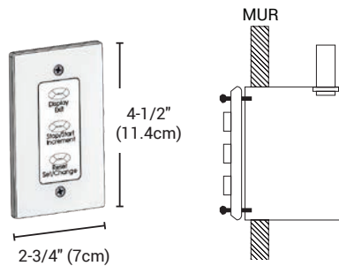
Commande du commutateur de temporisation
